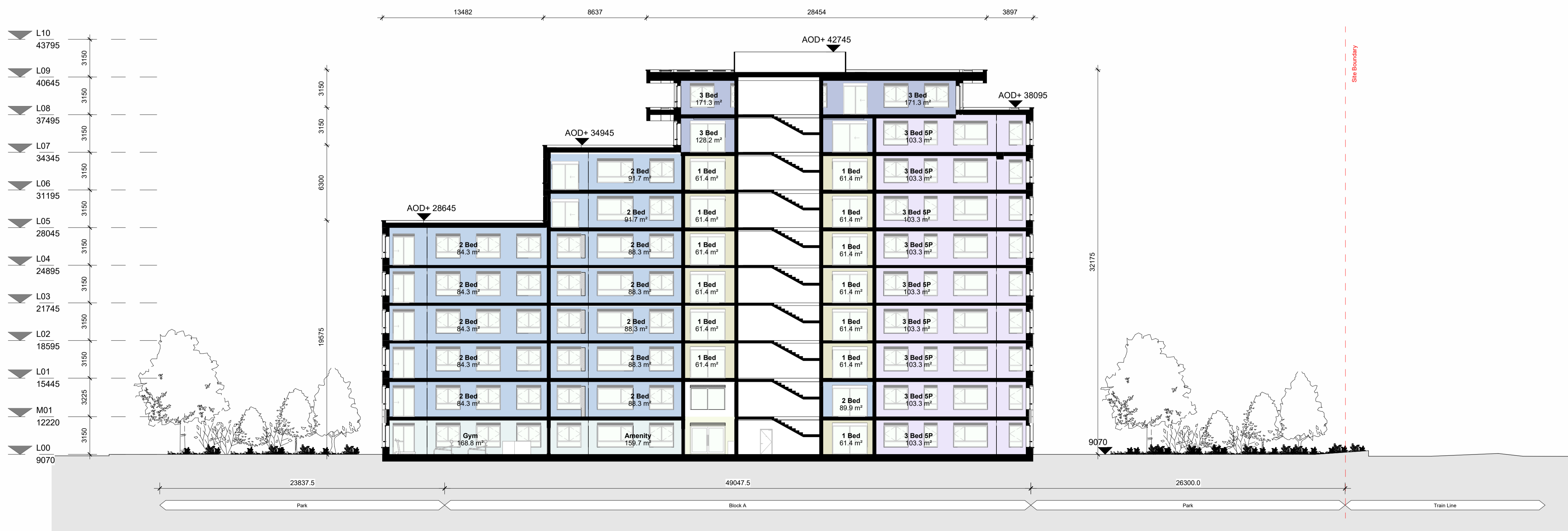
Block A Section DD 1 : 200
