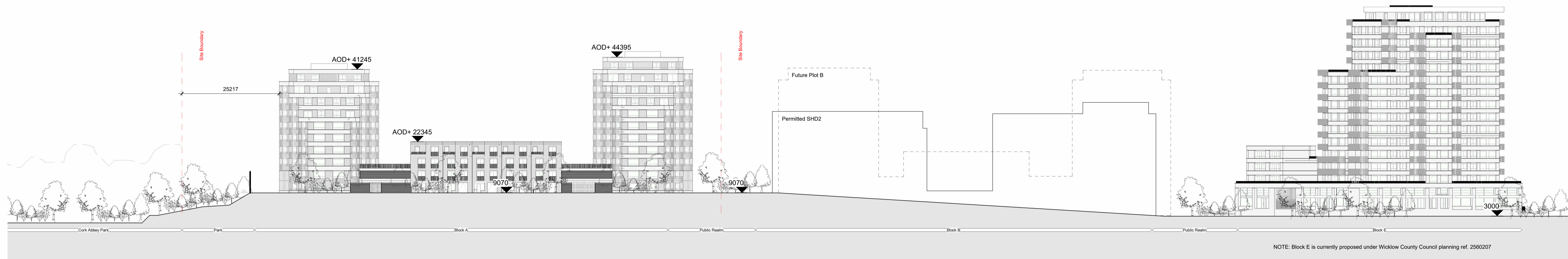
Site Elevation 02 1:500
